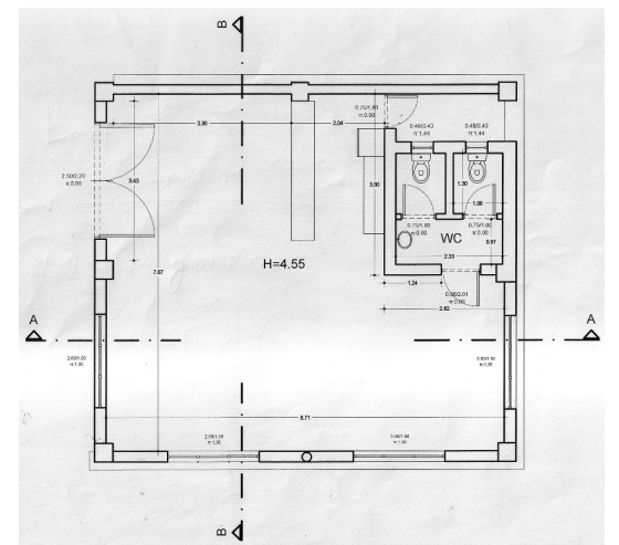
Κάτοψη
